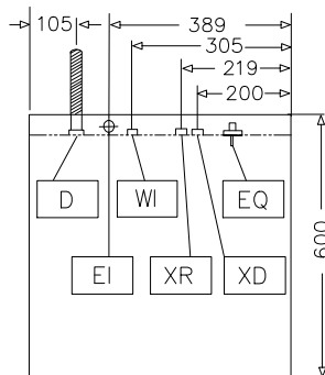
上视图 TOP-VIEW
